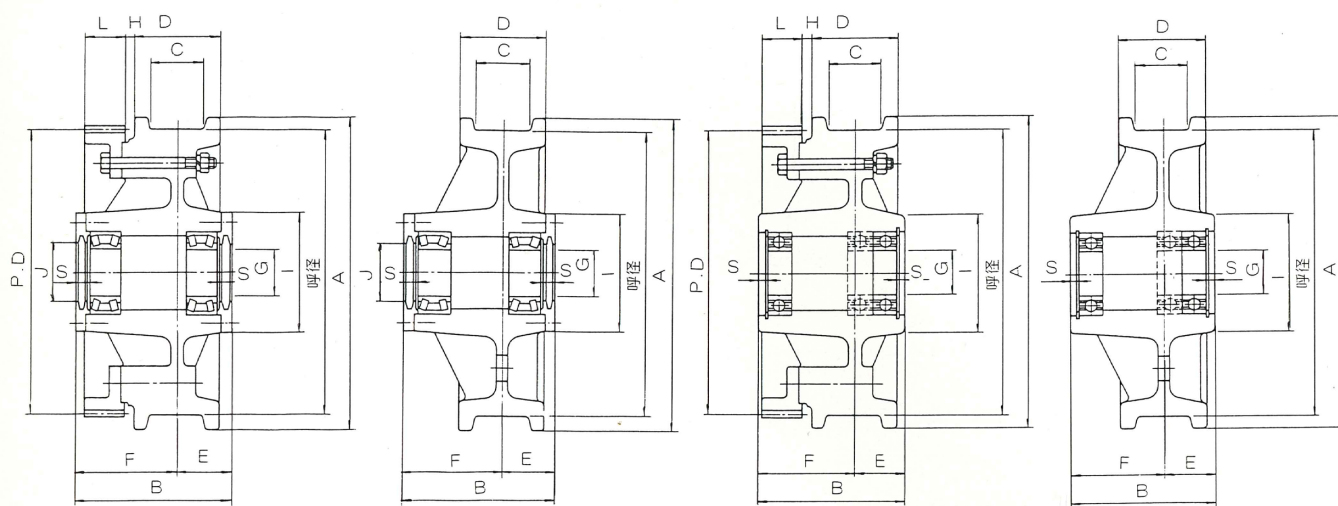
駆動車A (車輪踏面巾C-60)
